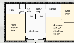
STUEPLAN DISPONIBEL BYGNING
